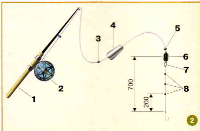
2. Снасть для ловли на квок: 1 – спиннинговое удилище; 2 – инерционная катушка; 3 и 5 – резиновые стопоры; 4 – пенопластовый скользящий поплавок; 6 – свинцовое скользящее грузило; 7 – стальное кольцо; 8 – подстроечные грузила.
