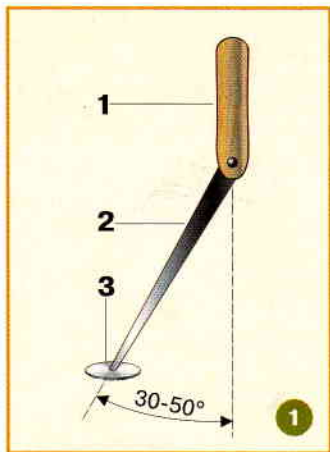
1. Квок для ловли сома: 1 – деревянная ручка; 2 – нож из стали или дюралюминия толщиной 0,8-2 мм; 3 – “пятачок” из стали или дюралюминия.
